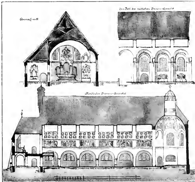
MOTTO ZWEISCHIFFIG. QUERSCHNITT, SÜDL. U. NÖRDL. INNENSICHT Nr. 15, Text S. VII—A, 2. u. 3. u. 4. u. 5.
